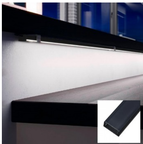
Perfil de aluminio de superficie para tira LED con difusor - 4 grapas - 2 tapas - 17x8mm - 2 metros
